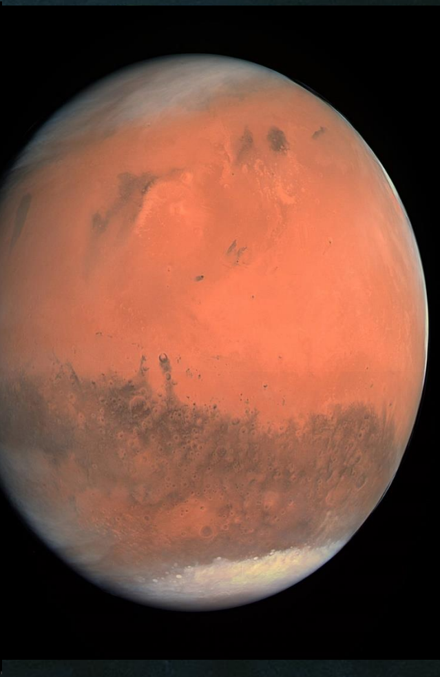
Mars
